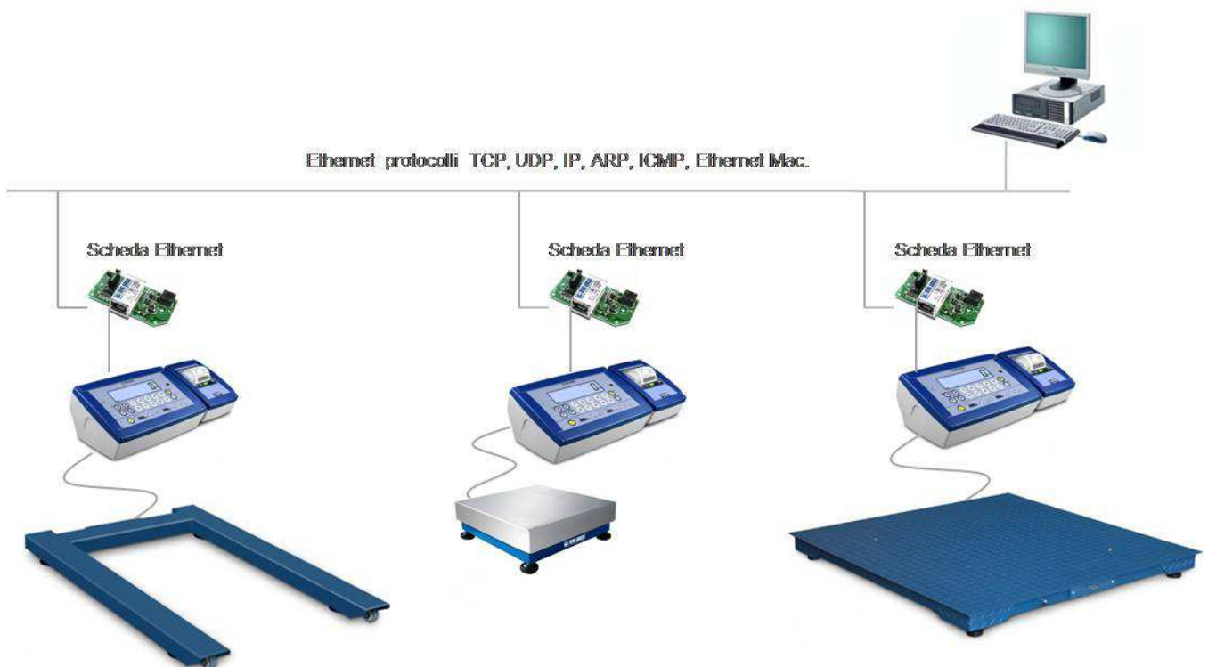
Fig. 1 Rete aziendale
